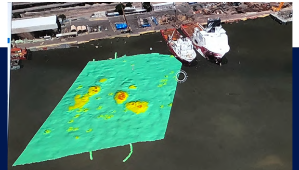
Batimetria do leito marinho no Porto de Santos
