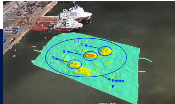
Batimetria do leito marinho no Porto de Santos
